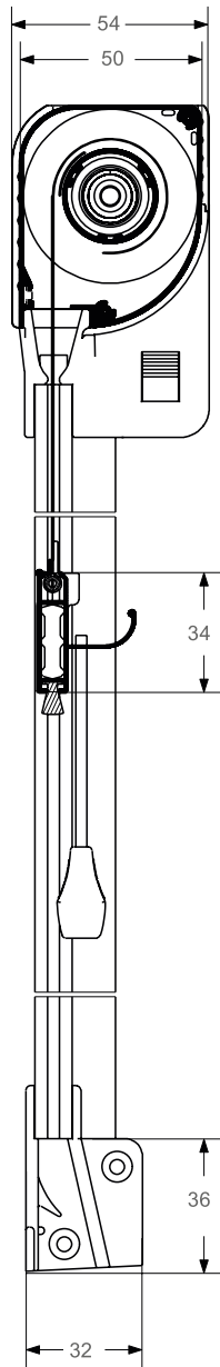
SEZ. VERTICALE
